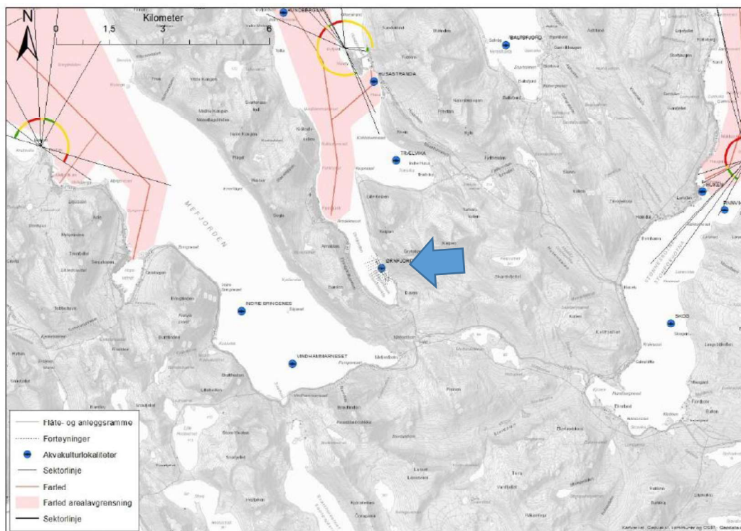
Figur 2 Viser sjøkart med anlegg, fortøyninger og lyktesektorer. Blå pil viser anlegget i Ørnfjordbotn. Anlegget vil ikke være til hinder for ferdsel på sjøen.
