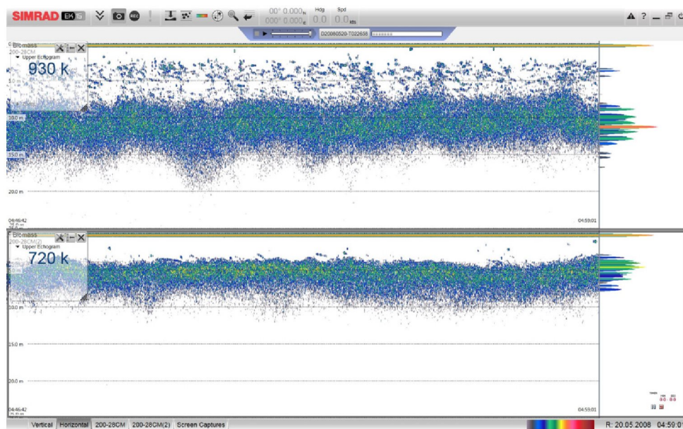
Figur 7 – Ekkoloddmålinger foretatt i Ventemerdd 2.
