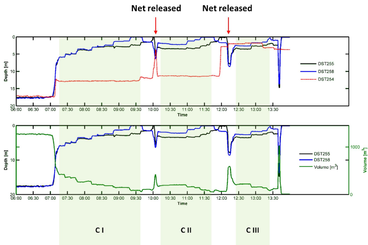
Figur 3 - Dybdemålinger og volumestimat i ventemerd. De grønne sonene (CI-CII) illustrerer tidsvinduerne for tre trengeoperasjoner i samme merd. Det ble tatt ut fisk fra start til slutt i CI og CII. Øverste figur - Rød kurve: notbunnens dybde i ikke-opplinet del; Blå og sort kurve: dybde av notbunn på to steder i delen av merden som lines opp. Nederste del – Blå og sort kurve: dybde av notbunn på to steder i delen av merden som lines opp. Grønn kurve: Estimert vannvolum i avkast under trenging.
