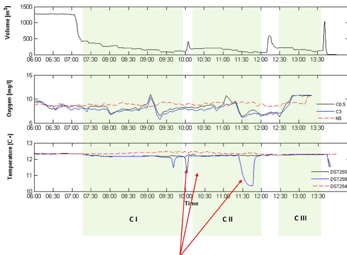
Figur 6 - Sammenstilling av volum av avkast, oksygennivå og temperatur under tre trengeprosesser (CI, CII og CIII) i Ventemerd 2. Med hensyn til oksygennivå, se Figur 5 for fargekoding av kurvene.
