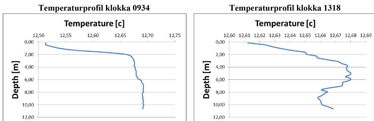
Figur 8 – Temperaturprofiler (temperatur ved ulike vanndybde) i ventemerdd 2 ved to tidspunkt (første og tredje trenging).
