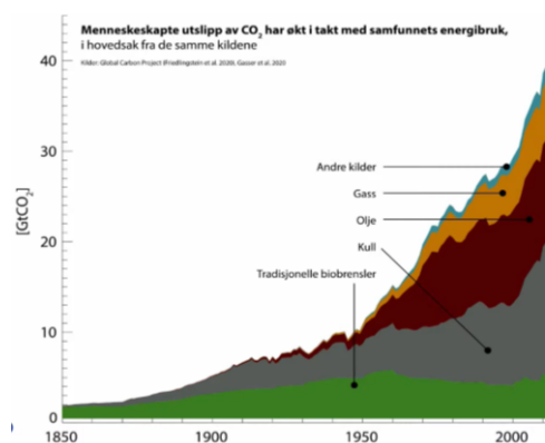
Figur 5 Menneskeskapte utslipp av CO 2 har økt i takt med samfunnets energibruk. Kilde: Cicero
