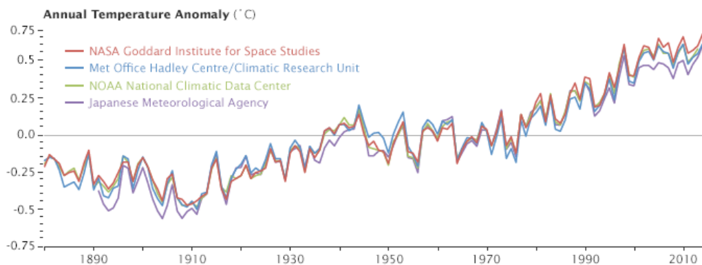
Figur 1 Temperaturutviklingen fra 1880 frem til 2014 i fire ulike tidsserier. Alle viser en tydelig oppvarming. Kilde: Cicero
