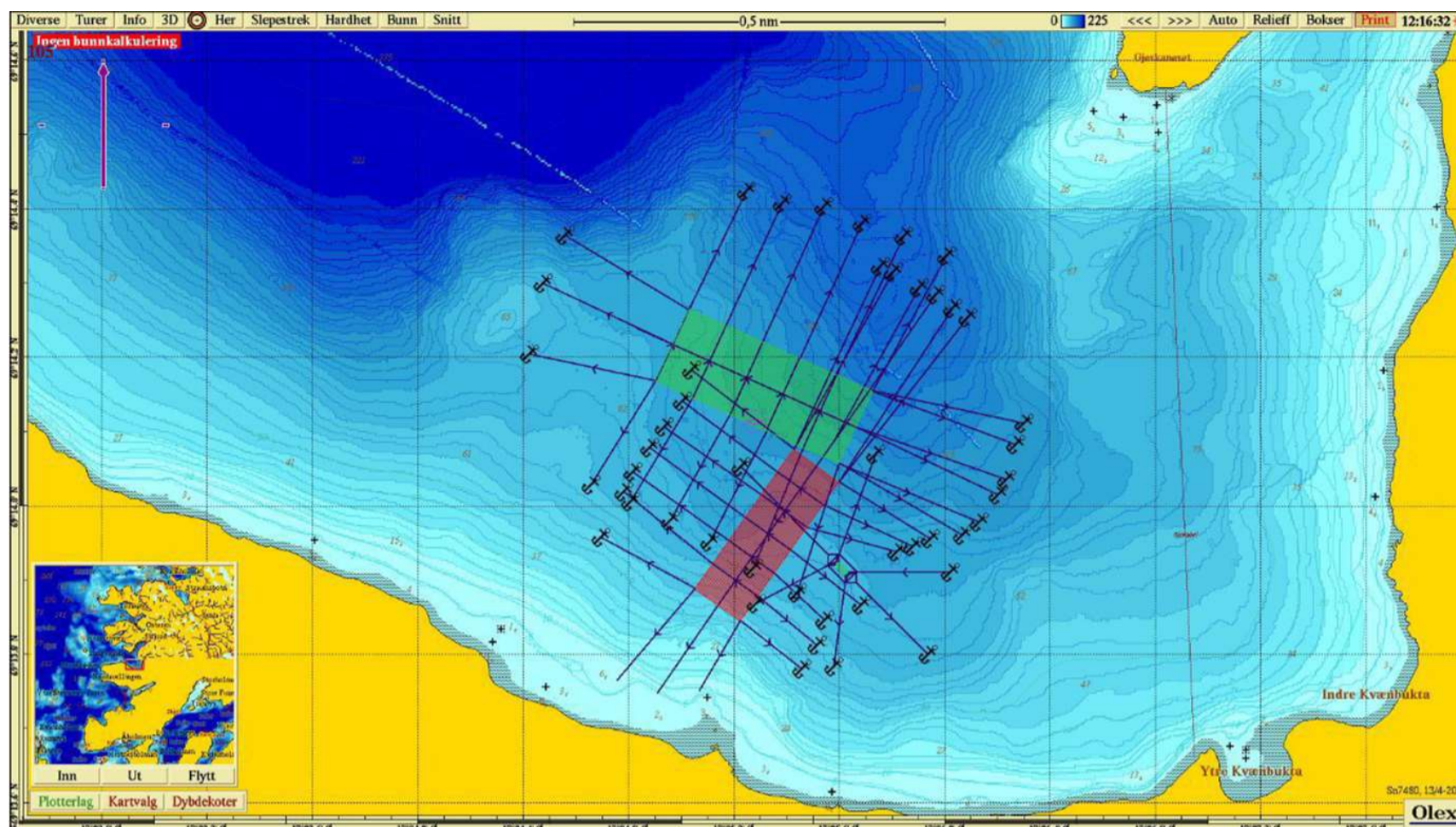
Figur 1: Rødt areal er dagens plassering av anlegget og grønt areal er omsøkte plassering. Som figuren viser, er omsøkte plassering lengre mot nord og rotert om lag 90 grader. Ny anleggsramme er ca. 500 x 200 meter og vil gi plass til 10 merder. Bilde hentet fra søknad.
